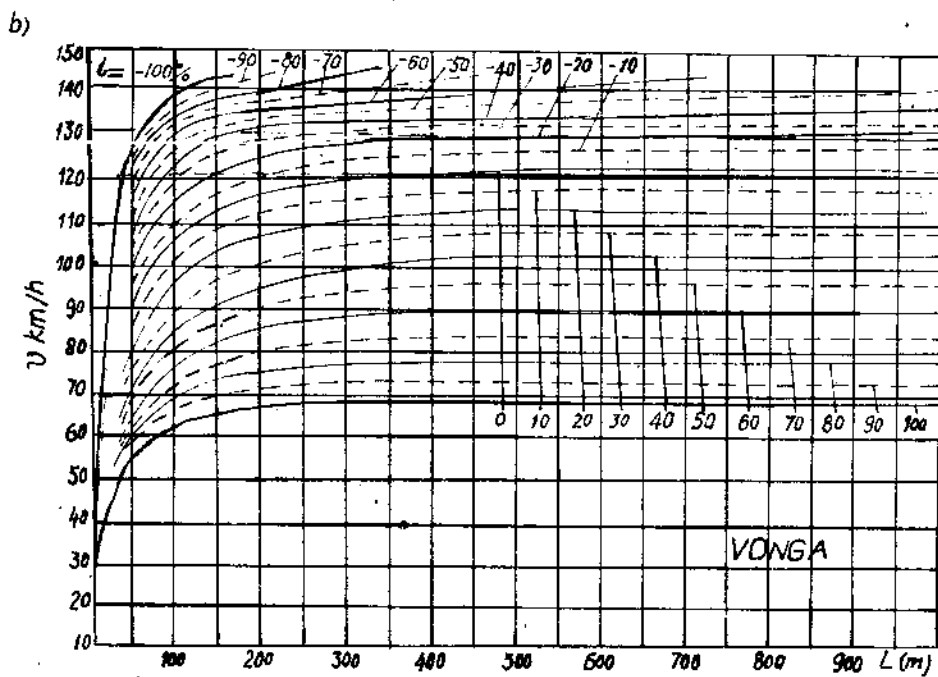
Hình 2-6. Đoạn tăng tốc của các xe con a - xe Motscovit ; b - xe Vonga.
