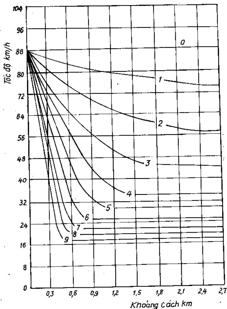
Hình 2-8b. Quan hệ tốc độ - hành trình của xe tải nặng điển hình (136 kG/mã lực), khi giảm tốc trên dốc dọc AASHTO 90.
