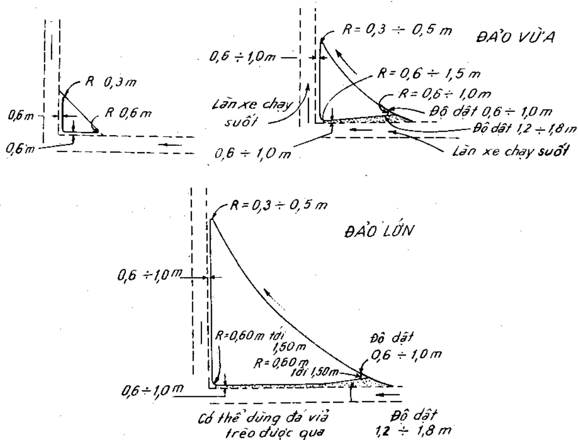
Hình 7-13. Chi tiết mép đảo có bao đá vữa, đường không có lề đường (có vỉa hè).
