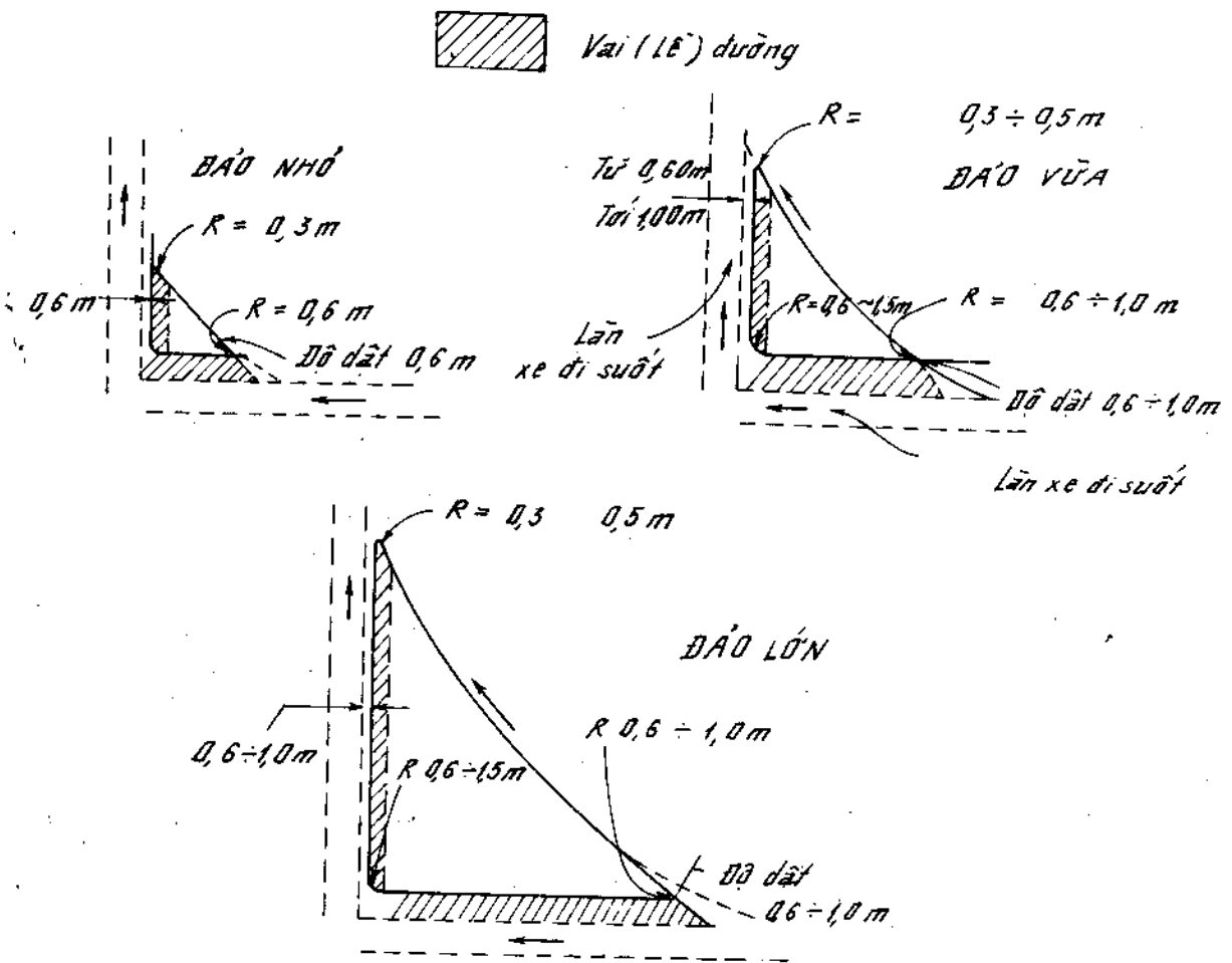
Hình 7-14. Chi tiết mép đảo có bao đá vĩa, đường có lề đường (không có vĩa hè)
